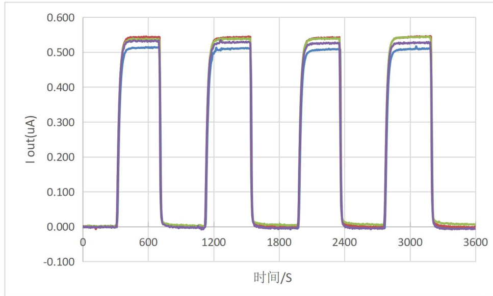
图 6 传感器对 500ppm 一氧化碳的重复性测试
