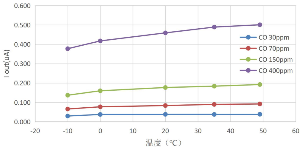
图 18 高低温运行试验
