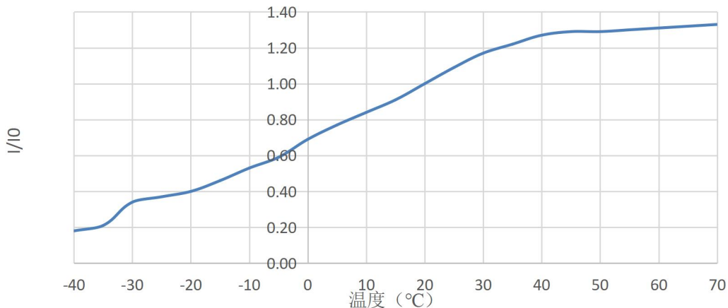
图 16 传感器温度补偿系数图示
