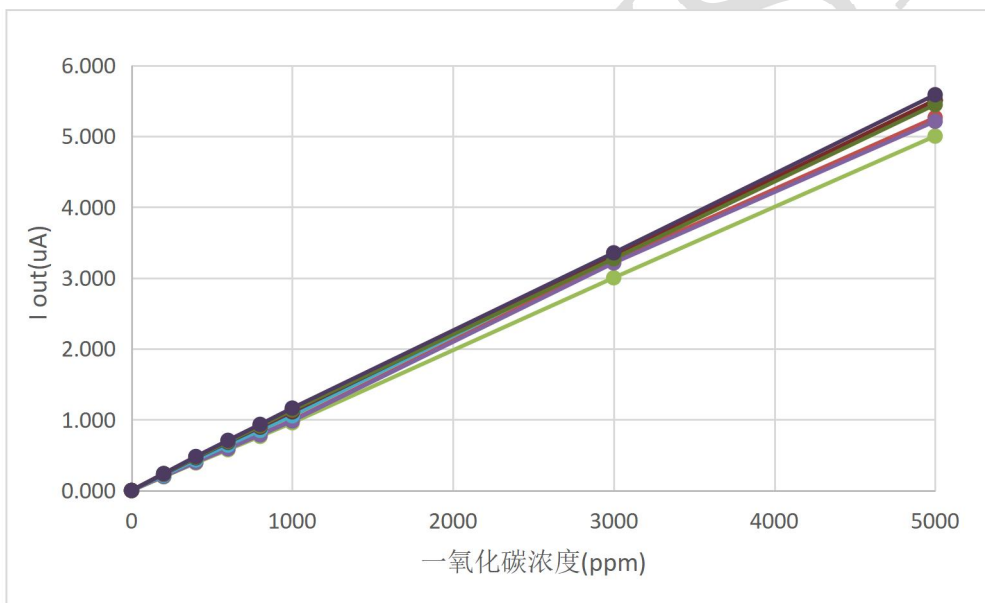
图 4 满量程线性图
