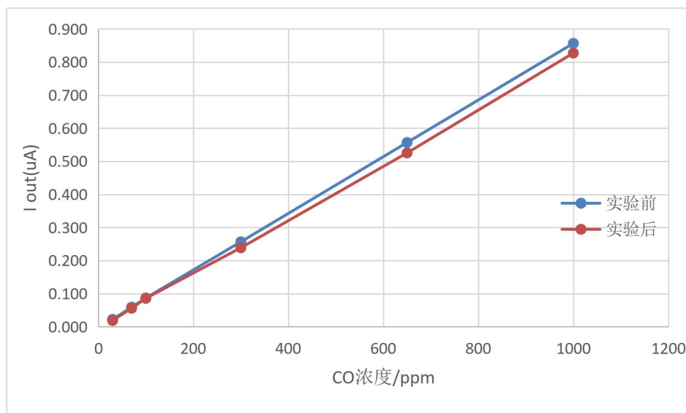
图 19 运输和储存试验前后变化
