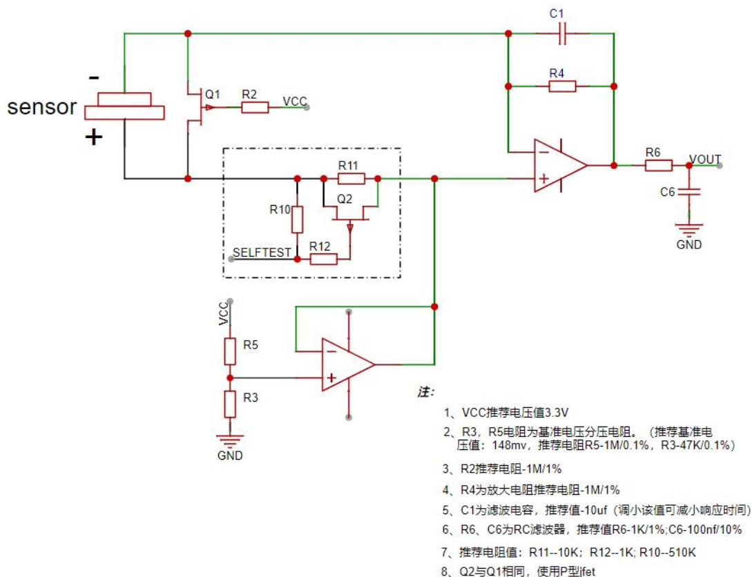
图 22 传感器电路示意图
