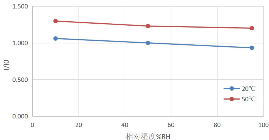
图 17 湿度影响
