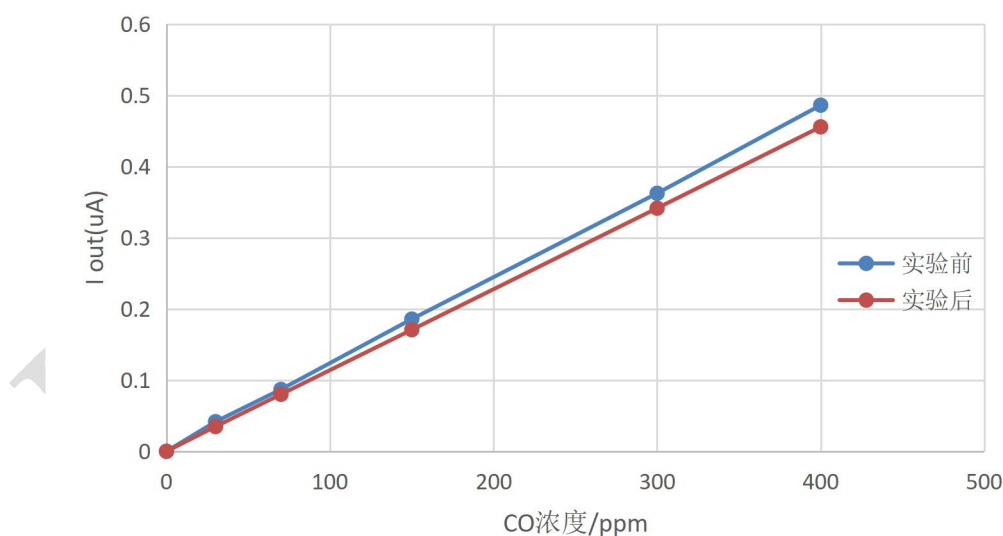
图 20 温度循环试验前后变化
