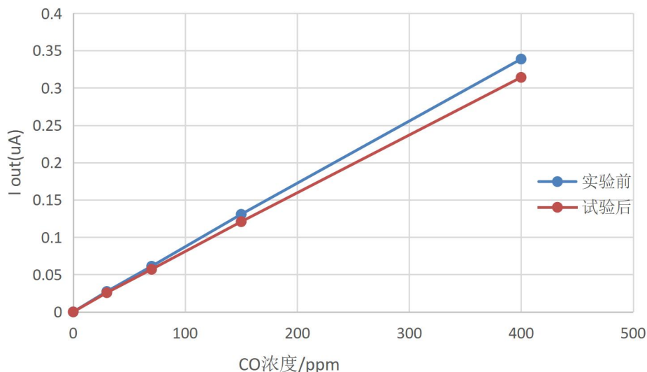
图 11 干扰气体试验前后测试变化
