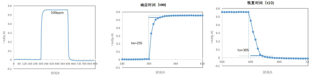
图 2 响应-恢复时间
