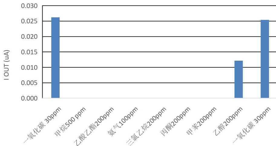
图10-干扰气体测试
