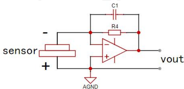
图 1 基本测试电路图
