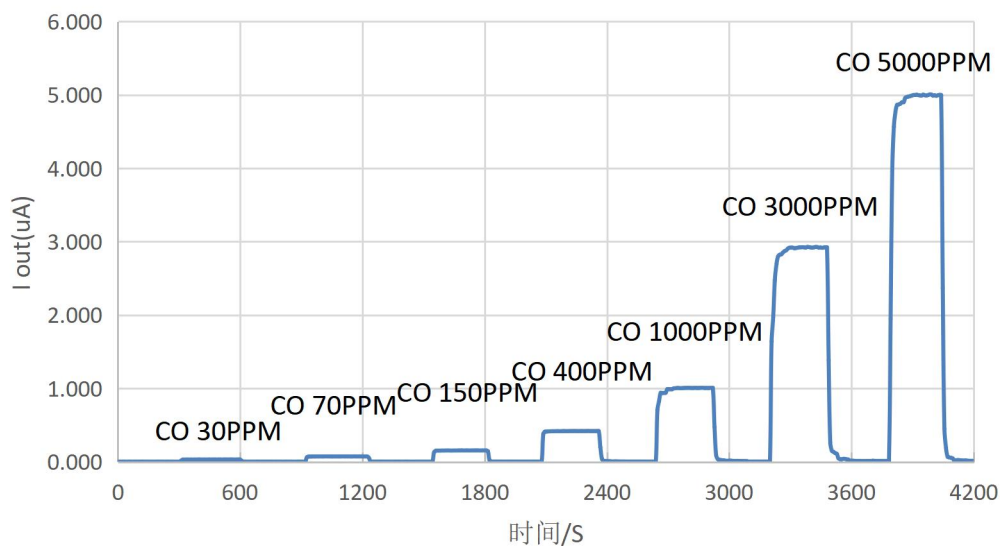
图 5 传感器响应特性
