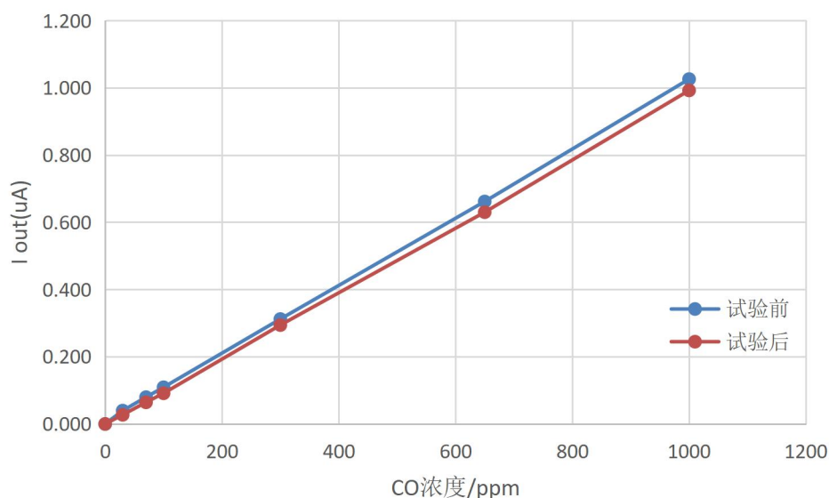
图 12 防腐性测试前后变化
